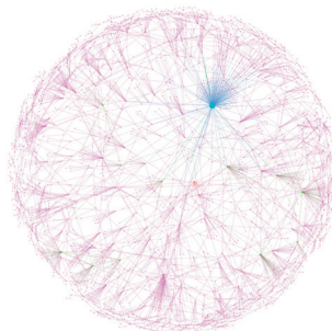
コンフィギュレーションモデルの巨大連結成分 Giant component of a configuration model
