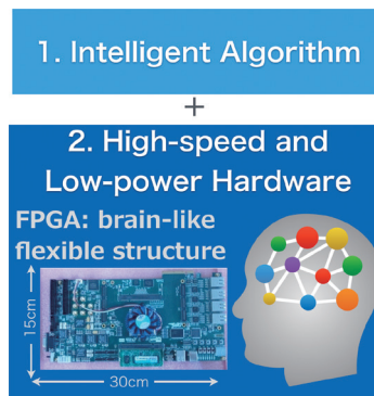
異なる計算領域からの大局的最適化 Global optimization across different computational domains
