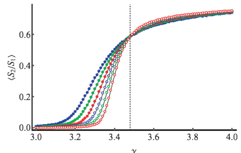
第1および第2連結成分の比による臨界点の特定 Finding critical point by the 1st and 2nd connected components
