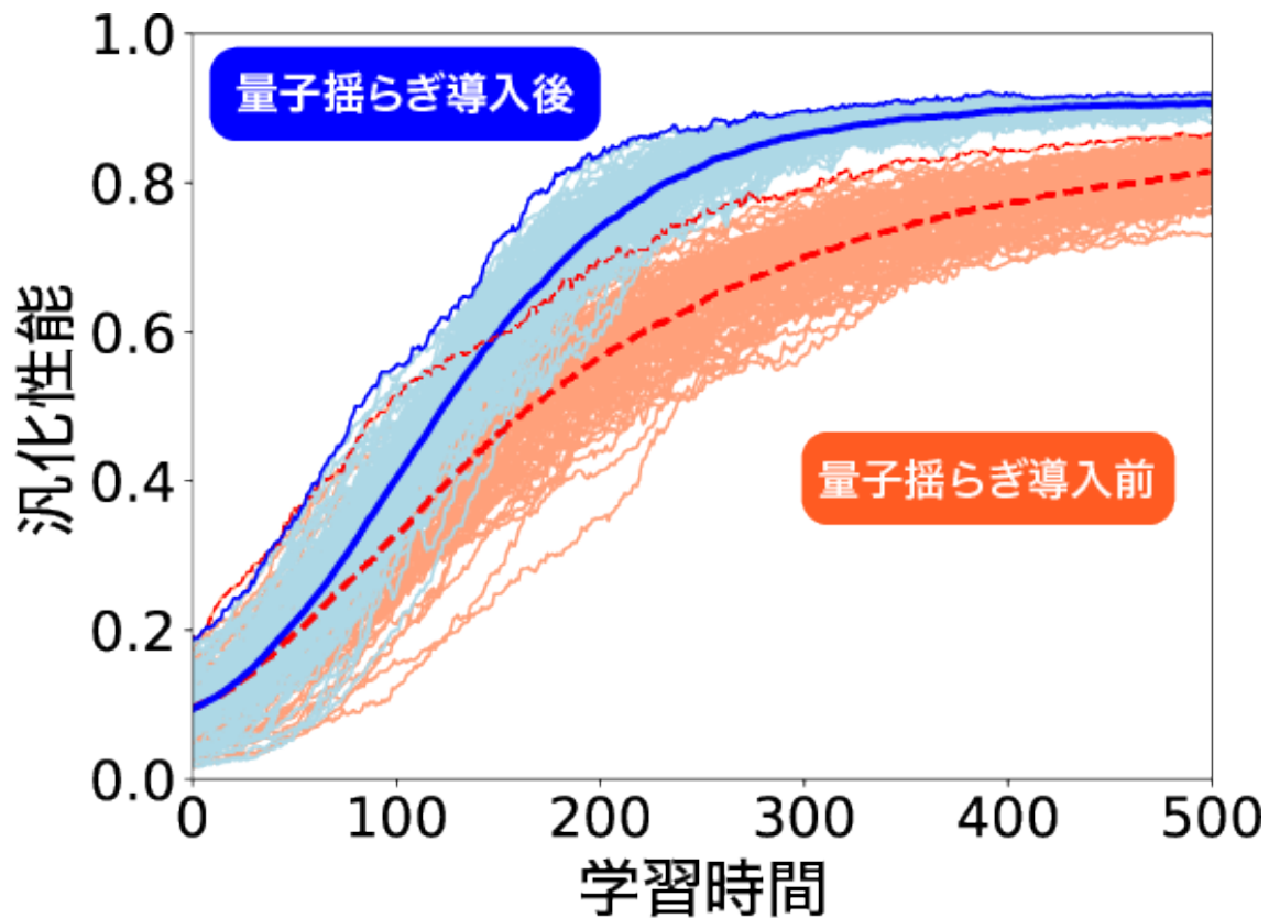
図 1:本研究成果で得られた量子揺らぎの効果例
